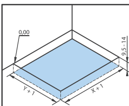
Vorbereitung montage
