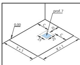
Vorbereitung montage
