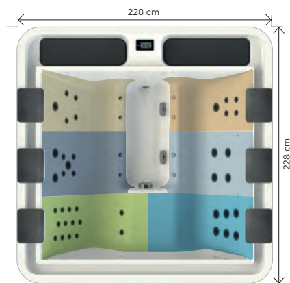
Hauteur 94 cm / Contenance : 1275 L
